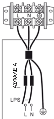
ΤΡΟΦΟΔΟΣΙΑ ΜΟΝΑΔΑΣ
