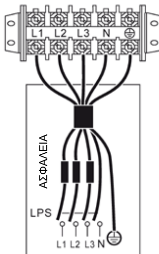
ΤΡΟΦΟΔΟΣΙΑ ΜΟΝΑΔΑΣ
